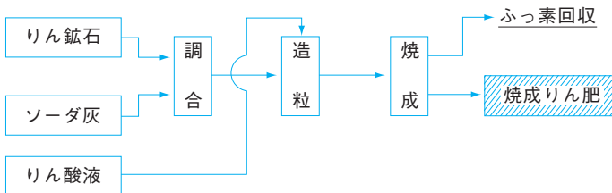
図一 1 焼成りん肥の製造工程
