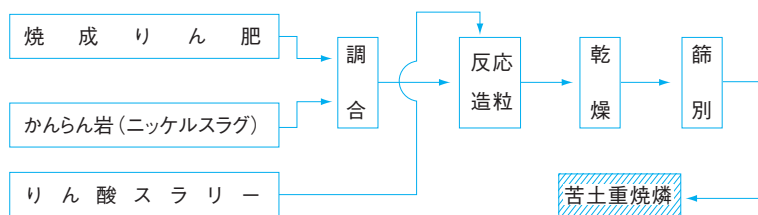
図－2 苦土重焼燐の製造工程
